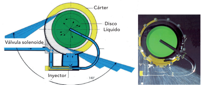
Fig. 19: Difusor centrífugo
